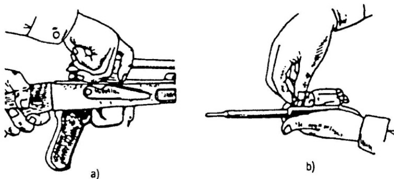
Hình 43: Tháo bệ khoá nòng và khoá nòng
