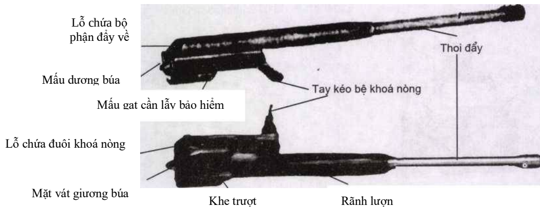
Hình 23: Bệ khoá nòng
