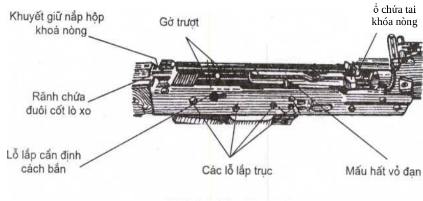
Hình 21: Hộp khoá nòng
