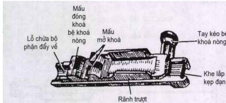
Hình 7: Bệ khoá nòng
