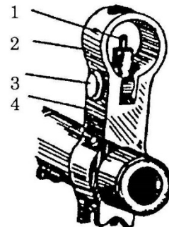
Hình 3: Bộ phận đầu ngắm
